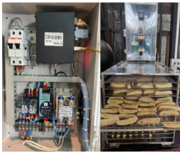
เครื่องอบแห้งด้วยลมร้อน ควบคุมด้วยสมาร์ทโฟน
